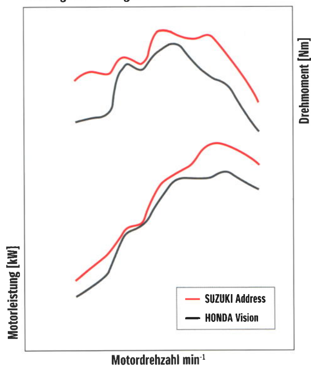
Leistungskurvenvergleich
